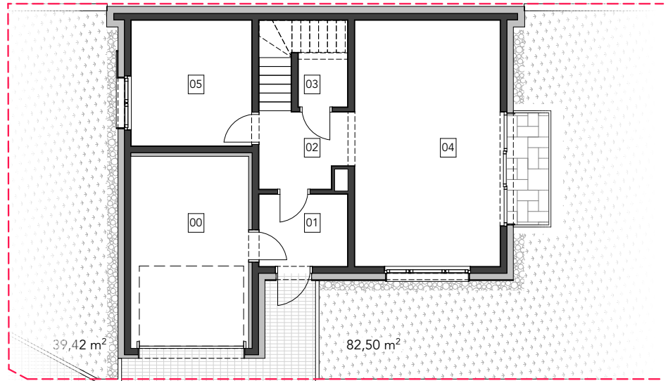
RZUT PARTERU
