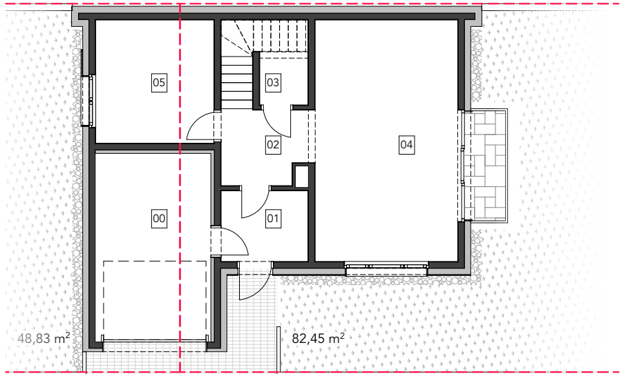
RZUT PARTERU
