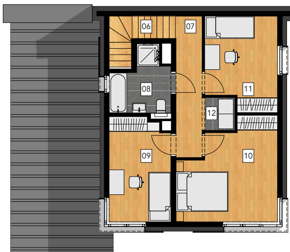
RZUT PIĘTRA
